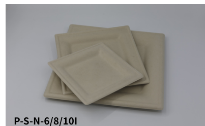
可降解餐盘 (6/8/10寸方盘) 底: 11g, 15g, 28g 盘箱规: 500pcs/箱 温度范围: -20°C~230°C 6-Inch: 160 \times 160 \times 10\text{mm} 8-Inch: 200 \times 200 \times 10\text{mm} 10-Inch: 260 \times 260 \times 15\text{mm}
